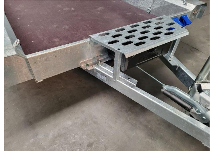
Vlemmix verschuifbare oprijplatenlengte 165cm 101.009.xxx Vloerhouderring gemonteerd. 321.001.116 Graafbak plateau, zonder kist 101.009.007 Kokers en roosters zijn 60mm i.p.v. 40mm. Roosters zijn smaller dus meer verticaal draagvermogen. Hier is geen meerprijs ten opzichte van de standaard klep.
